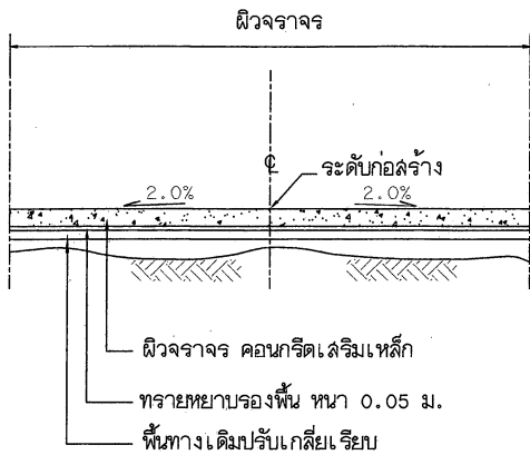
รูปตัดแสดงโครงสร้างถนนคอนกรีตเสริมเหล็ก
