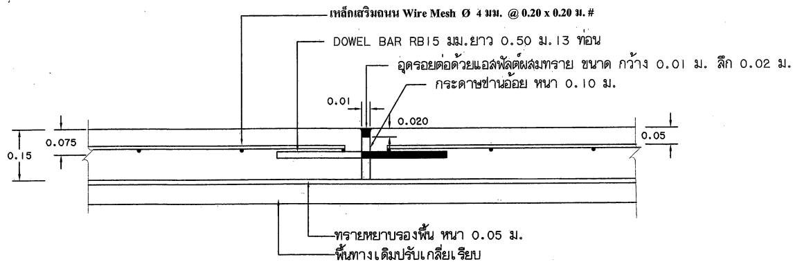
ขยายรอยต่อ EXPANSION JOINT NOT TO SCALE
